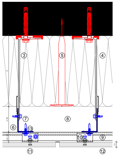
Horizontalschnitt / horizontal section
