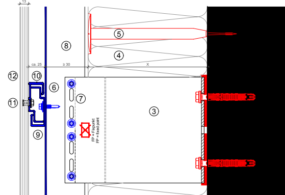
Vertikalschnitt-Fixpunkt / vertical section-fixed point
