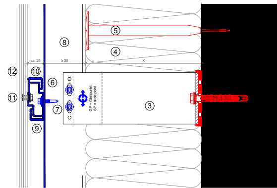
Vertikalschnitt-Fixpunkt / vertical section-fixed point
