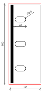
Dübel/ anchor
