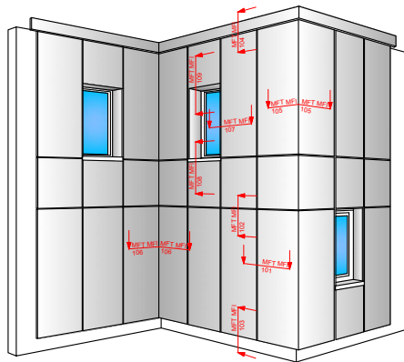
Fassadenansicht / view of cladding
